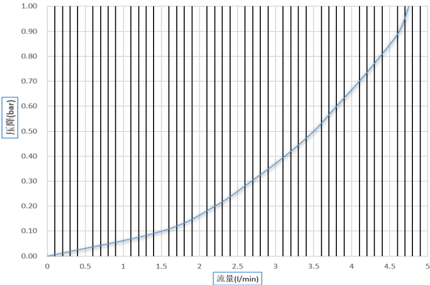
MDC04 流量曲线
